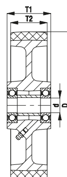
cuscinetto a sfere
